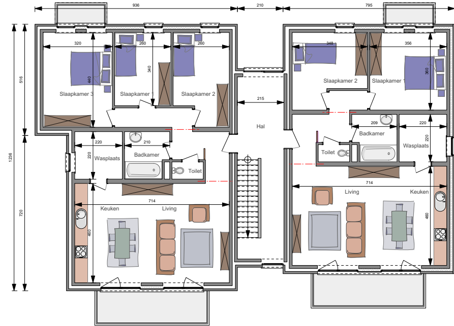
VERDIEPING 1
