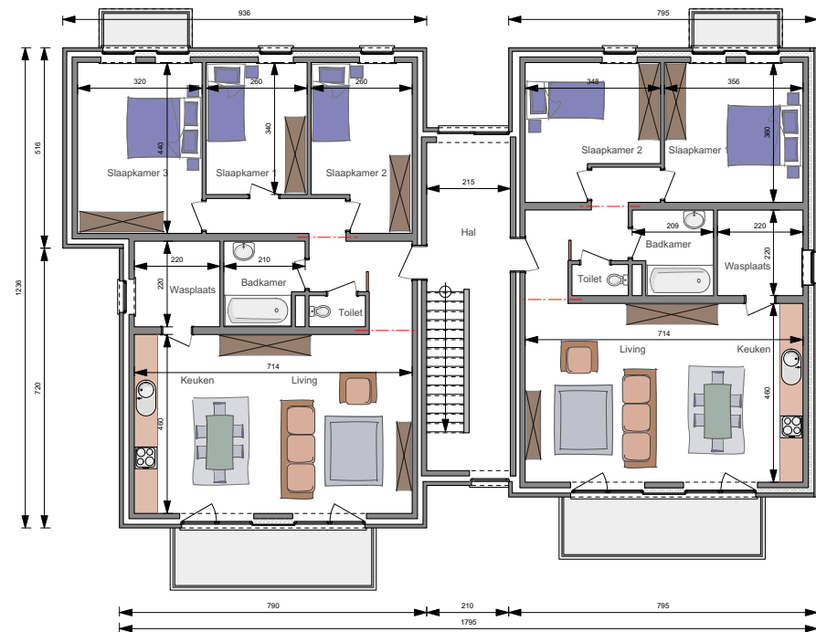
VERDIEPING 2
